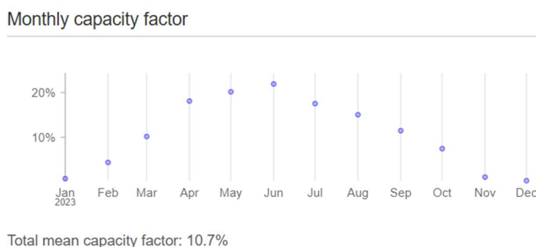
Kuva 11. Kuukausittainen aurinkovoiman kapasiteettikertoimen vaihtelu, Seinäjoen seutukunta.
