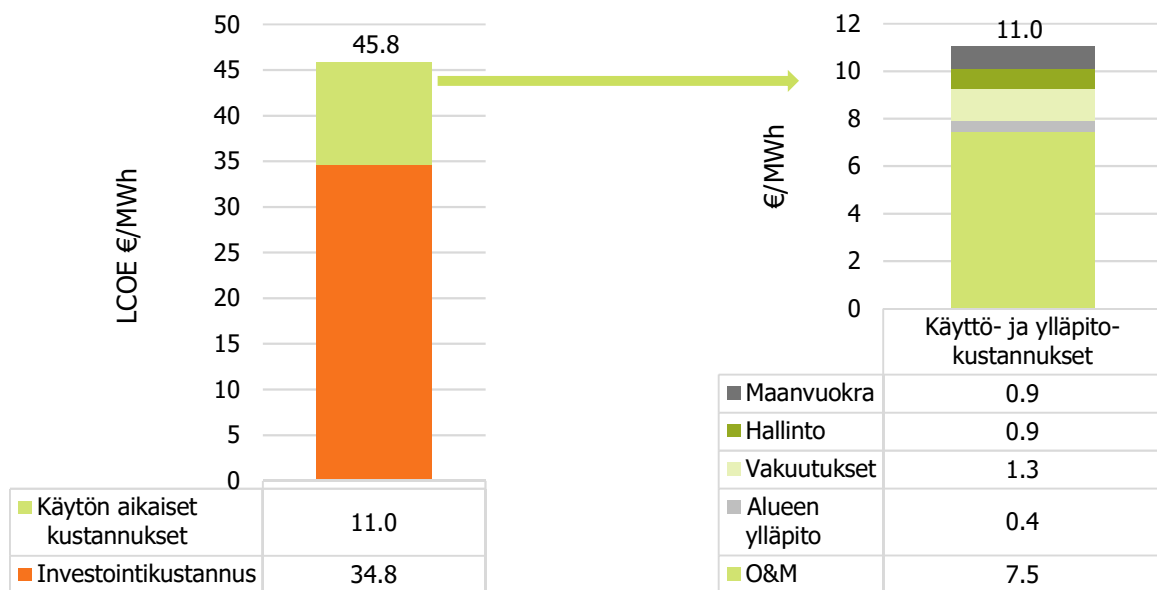
Kuva 25. Oikealla tuulivoiman tuotantokustannus jaoteltuna investointi- ja käytön aikaisiin kustannuksiin. Oikealla käytön aikaisten kustannusten jakautuminen.
